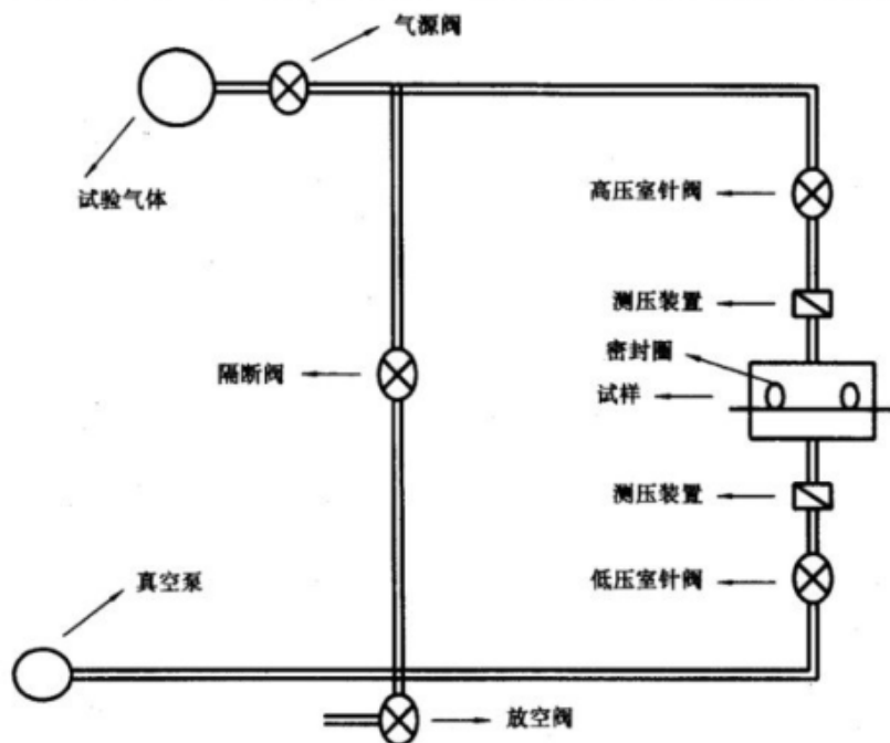
图 1 透气仪
